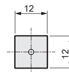
단면 AA
